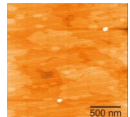
InAs-Quantenpunkte auf einer GaAs(100)-Oberfläche
