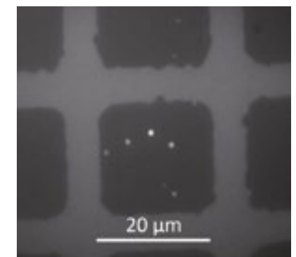
Kryogene Lokalisierung von einzelnen Quantenpunkten in Diodenstrukturen. Die hellen Punkte im Bild sind Photolumineszenz einzelner Quantenlichtquellen.
