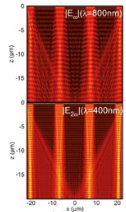
Simulation der elektrischen Felder in dem Bauelement zur Frequenzkonversion.
