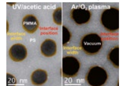
Numerisch unterstützte Präzisionsmessungen der Geometrie von unterschiedlich prozessierten Nanomasken aus einem Block-Copolymer
