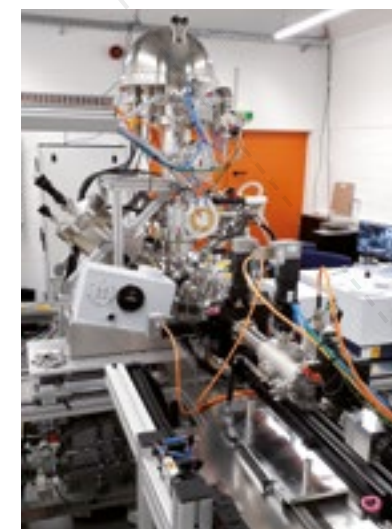
In 2021/22 etablierter Aufbau zur Analyse von Grenzflächenprozessen mittels Near-Ambient-Pressure XPS (NAP-XPS)
