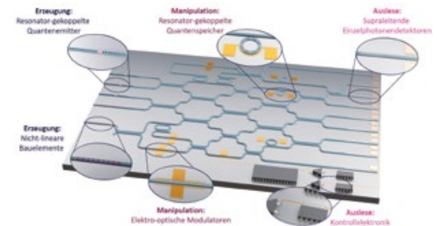
Schematische Darstellung eines quantenphotonischen integrierten Schaltkreises für die Erzeugung, Manipulation und Auslese von Quantenzuständen (Qubits). Wesentliche Bauelemente sind in den Einblendungen hervorgehoben. (© Klaus Jöns)
