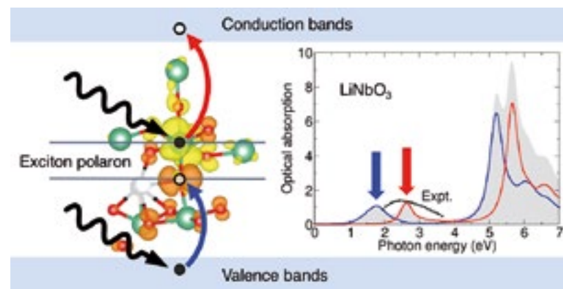
Optische Übergänge von defektgebundenen Exziton-Polaronen in Lithiumniobat und berechnete Beiträge zur transienten Absorption
