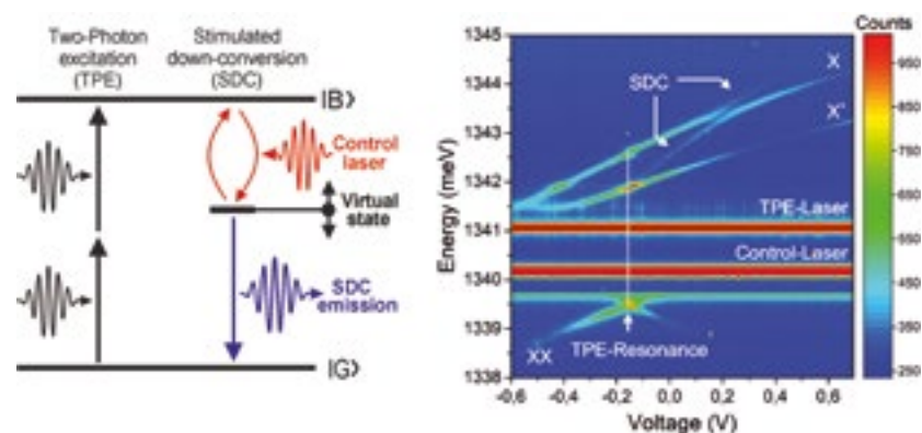
Links: Schematische Darstellung der stimulierten Abwärtskonversion (SDC) im Quantenpunkt zur Erzeugung einer abstimmbaren Einzelphotonenemission. Rechts: Experimentelle Realisierung, aus B. Jonas et al., Nat. Comm. 13(1), 1387 (2022)
