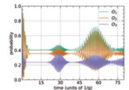
„Collapse and revival dynamics“ der Besetzungen eines Dreiniveausystems, das mit 2 Quantenlichtmoden wechselwirkt
