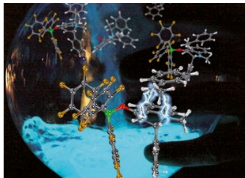
Sigmatrope [1,5] Kohlenstoffverschiebung
