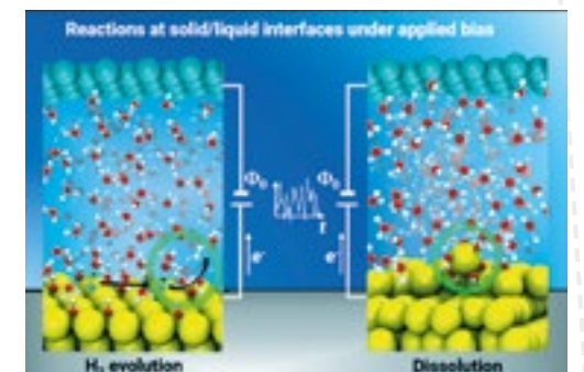
Reaktionen an Fest-/Flüssig Grenzflächen unter realistischen Bedingungen und angelegter Spannung: (links) Wasserstoffentwicklung und (rechts) Mg Auflösung unter anodischen Bedingungen. Die Spannung wird zwischen zwei Elektroden angelegt (gelbe und türkisfarbene Atome), zwischen denen sich Wasser befindet (O: rot, H: weiß). (Foto: Dr. Mira Todorova)
