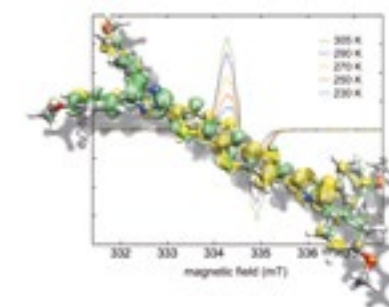
Open-Shell Chinoid mit thermisch anregbarem Singulett-Triplett-Übergang
