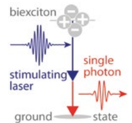
Erzeugung eines einzelnen Lichtteilchens mit optisch kontrollierbaren Eigenschaften. Zu Nature Communications 13, 1387 (2022)
