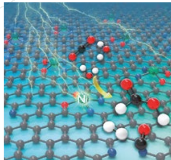
Grafische Darstellung der Umwandlung von CO 2 und H 2 O in H 2 und Formaldehyd über einer nickeldotierten Kohlenstoffschicht
