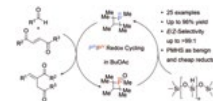
Nachhaltige Variante der basenfreien katalytischen Wittig-Reaktion
