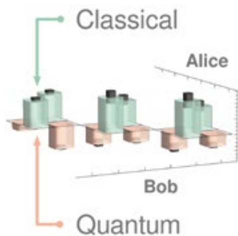
Erste Rekonstruktion einer Verbundwahrscheinlichkeit mit negativen Beiträgen als Nachweis von Quantenverschränkung, gemeinsam mit AG Silberhorn.
