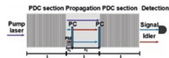
Zweifarbige integriertes SU(1,1)-Interferometer
